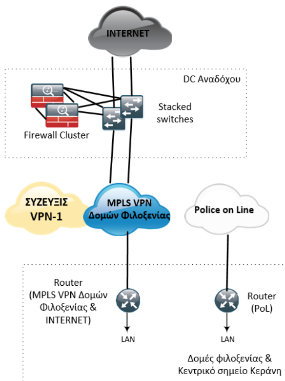
Εικόνα 1. Αρχιτεκτονική υλοποίησης δικτύου
